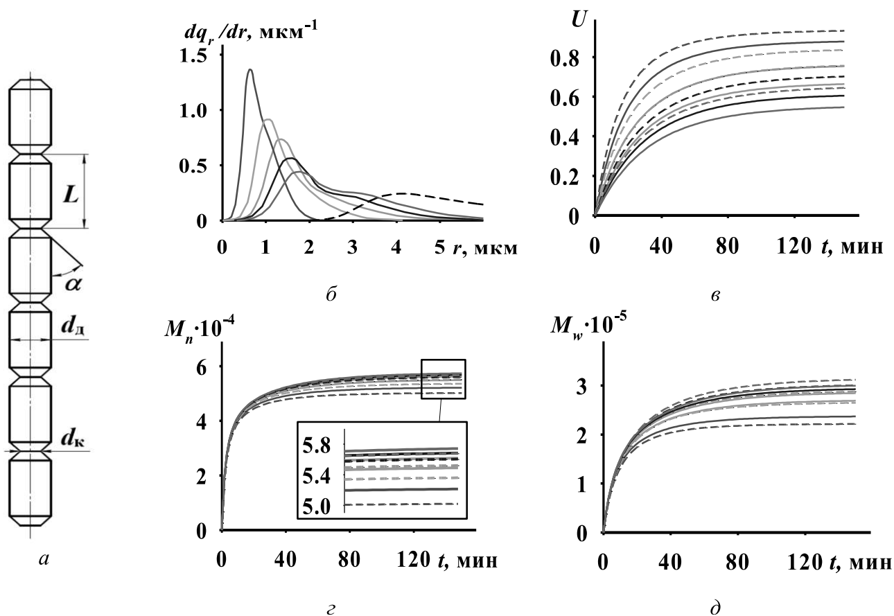
Рис. 3. Продольное сечение трубчатого турбулентного аппарата диффузор-конфузорной конструкции (а), распределения частиц каталитической системы \text{TiCl}_4 + \text{Al}(\text{изо-С}_4\text{Н}_9)_3 по эквивалентному радиусу до (пунктирная линия) и после (сплошные линии) пропускания реакционной смеси гомополимеризации бутадиена через трубчатый турбулентный аппарат диффузор-конфузорной конструкции (б), временные зависимости выхода сополимера U (в), среднечисленной M_n (з) и среднемассовой M_w (д) молекулярных масс сополимера в сополимеризации бутадиена и изопрена в присутствии каталитической системы \text{TiCl}_4 + \text{Al}(\text{изо-С}_4\text{Н}_9)_3 , проводимой по способу 2; d_d = 24 мм, d_d/d_k = 8/3 (красный), 8/4 (оранжевый), 8/5 (зеленый), 8/6 (синий), 8/7 (пурпурный), L = 48 мм, \alpha = 45^\circ , число секций – 6, v = 0.9 м/с; q = 0.76 (сплошные линии на в-д), q = 0.85 (пунктирные линии на в-д)
